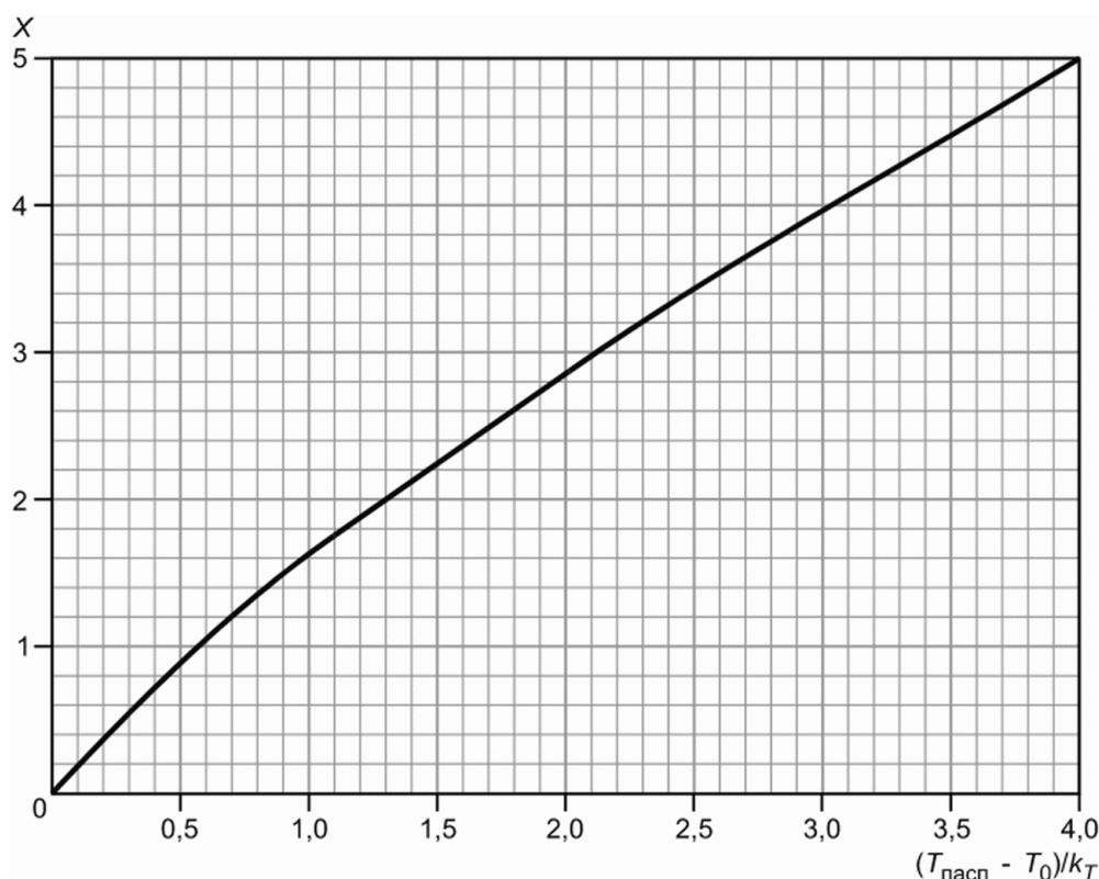
Рисунок В.2 - График для интерполяционного определения времени активации спринклерного оросителя при термическом
